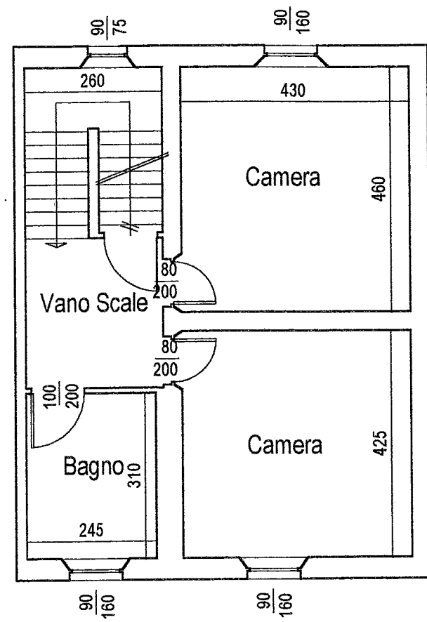
Piano Primo Stato Modificato
