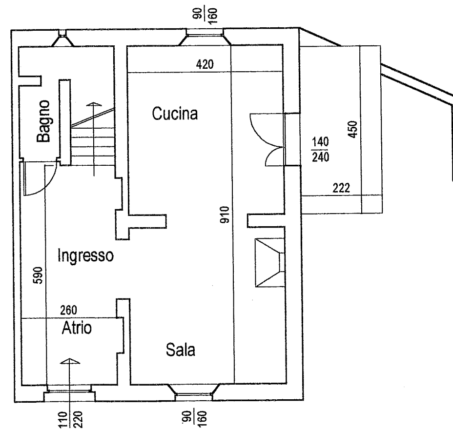
Piano Terra: Stato Modificato
